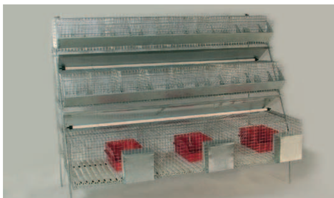
Art. 05 cm 208 x 94 x 145 h Gabbia mista per riproduzione ed ingrasso, con 3 box fattrici e 16 box per l'ingrasso
