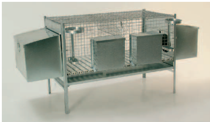
Art. 09 cm 100 x 50 x 65 h Gabbia smontabile per fattrici conigli a 2 cove
