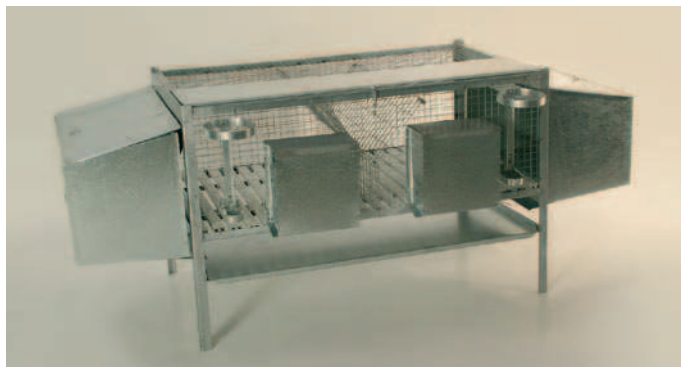
Art. 11 cm 100 x 60 x 65 h Gabbia fissa per fattrici conigli a 2 cove
