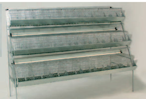
Art. 06/c cm 208 x 94 x 145 h Gabbia per l'ingrasso con 24 box (cm. 25 x 36), costruita interamente in rete a doppia zincatura, fondo in plastica
