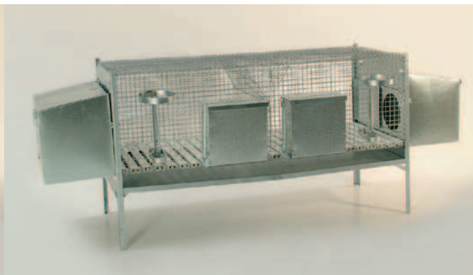
Art. 10 cm 120 x 50 x 65 h Gabbia smontabile antitopo per fattrici conigli a 2 cove
