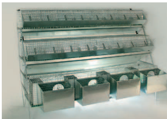
Art. 06 cm 208 x 94 x 145 h Gabbia mista per riproduzione ed ingrasso, con 4 box fattrici e 16 box per l'ingrasso, fondo in plastica
